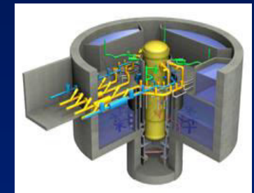
ESBWR
