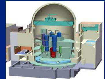
USAPWR
